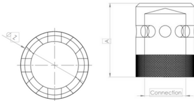
Dimensioni dell'ugello
